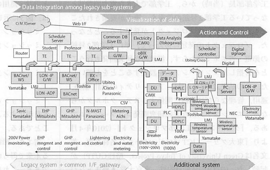
図4 工学部2号館システム概要図
